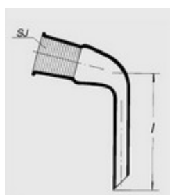
Předloha destilační - (alonž), s NZ typ 8179
