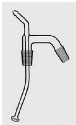
Nástavec na přehánění vodní parou typ 8154
