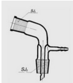
Předloha destilační - (alonž), s olivkou a s NZ typ 8180
