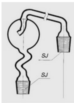
Nástavec destilační - s lapačem kapek, s NZ typ 8147
