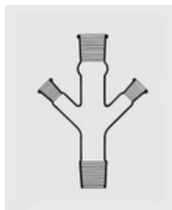
Spojkové díly - sestavené do řetězce typ 8223, 8222
