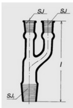
Nástavec destilační - se svislou odbočkou typ 8233
