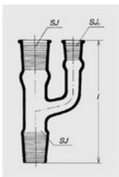
Nástavec destilační - se svislou odbočkou typ 8232
