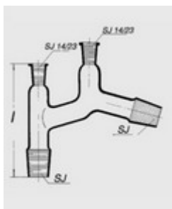
Nástavec destilační dle Claisena - s NZ typ 8173
