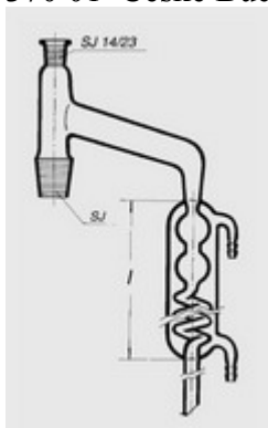
Nástavec destilační - s NZ se spirálovým chladičem typ 8176
