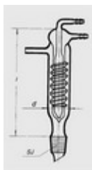
Chladič zpětný - šroubový s bočním přívodem typ 8267
