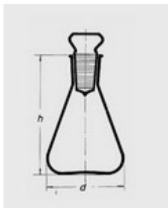
Baňka na stanovení jodového čísla - se skleněnou zátkou typ 8481
