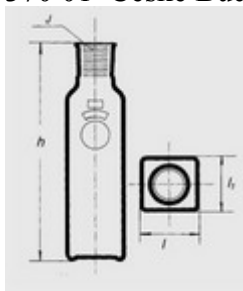
Baňka kultivační - dle Blacka typ 3120
