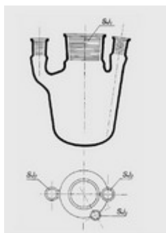
Baňka sulfonační - se 3 postranními tubusy typ 8022
