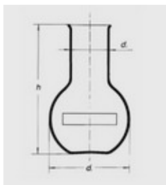
Baňka titrační - ploché dno, širokohrdlá, vyhnutý okraj typ 18
