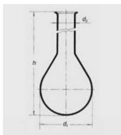
Baňka mineralizační - podle Kjeldahla typ 51
