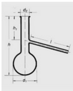
Baňka frakční - s trubicí natavenou dole typ 41/A
