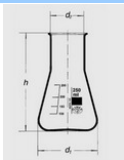
Baňka kuželová dle Erlenmeyera - širokohrdlá typ 25
