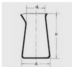
Kádinka podle Philipse - nízký tvar typ 161
